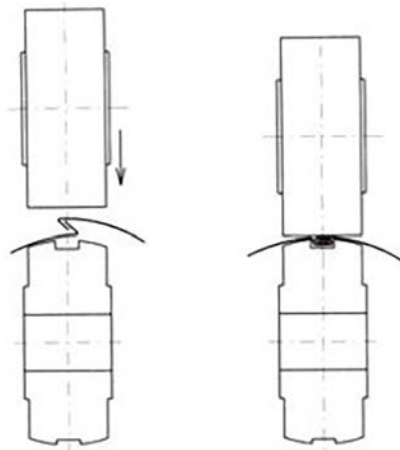
ABB.: SKIZZE DRÜCKPOSITION
